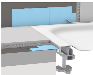
Dichtsystem Für Badewanne und Dusche - flexibel und schnell zu installieren.
