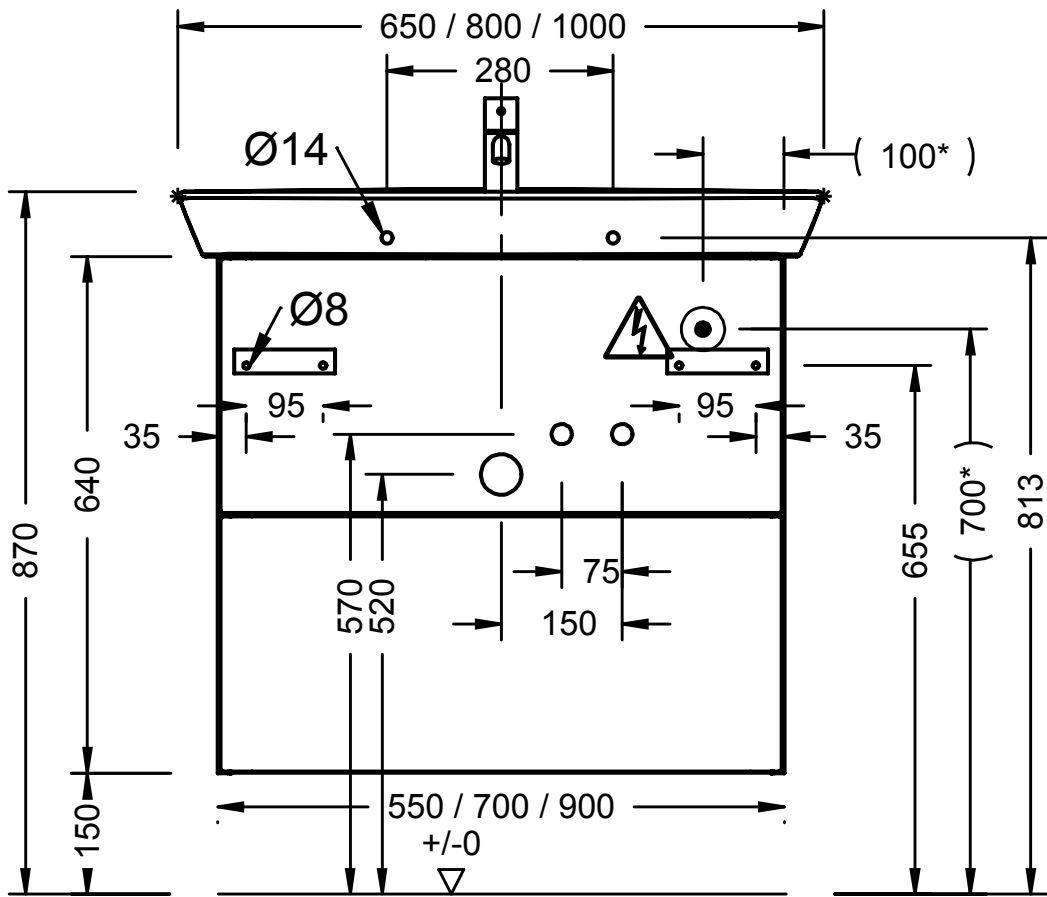
SFEN065, 080, 100 (*) SFEY065, 080, 100
