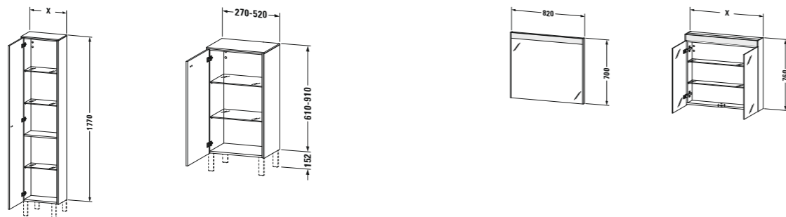
Hochschränke Tall cabinets Armarios altos
