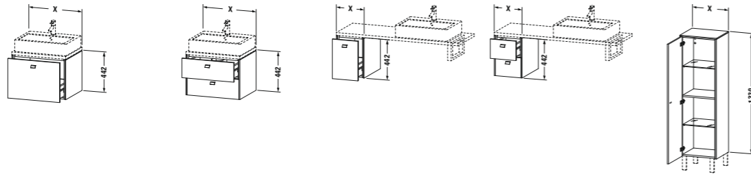
Waschtischunterbauten für Konsole Vanity units wall-mounted for console Muebles para lavabo para encimera
