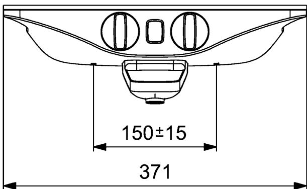
Produktzeichnung
