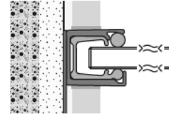
Einbausituation B Montage auf Putz
