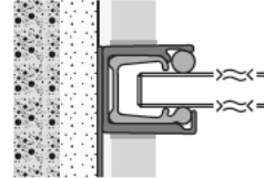
Einbausituation B Montage auf Putz
