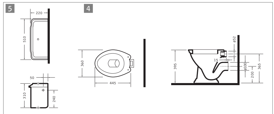
4 112.61.000 Tiefspülklosett, Abgang außen waagrecht
