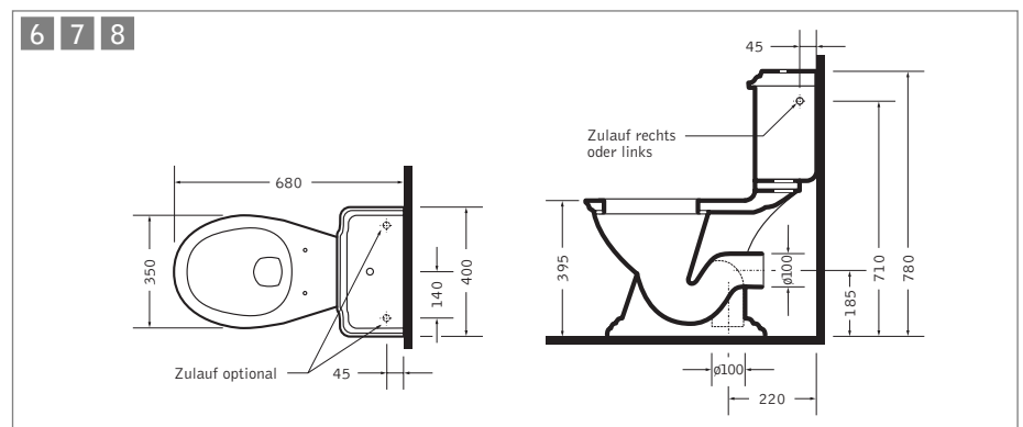
7 112.67.000 Tiefspülklosett zu Klosettkombination Abgang außen waagrecht
