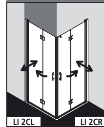
Ecke: LI 2CR und LI 2CL
