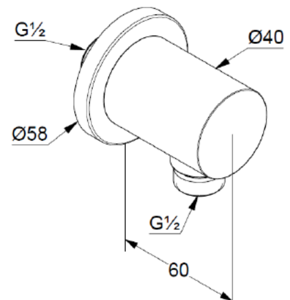
Maßzeichnung
