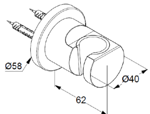
Maßzeichnung
