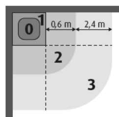
Bereichseinteilung Raum mit Dusche
